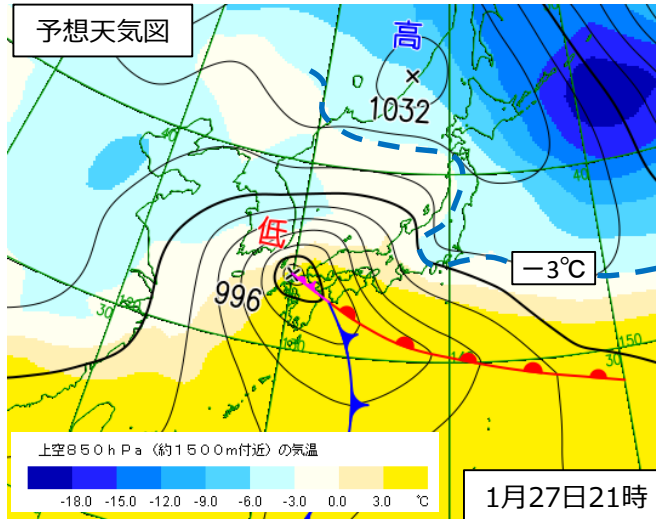
地上天気図と上空約1500mの気温（予想） 27日21時
